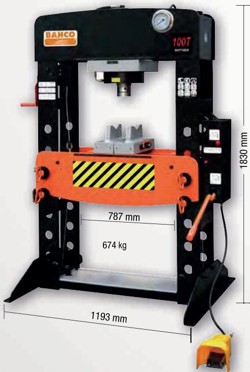
Presse hydropneumatique 100T
