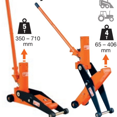
BH1S45 Nůžkový zvedák
